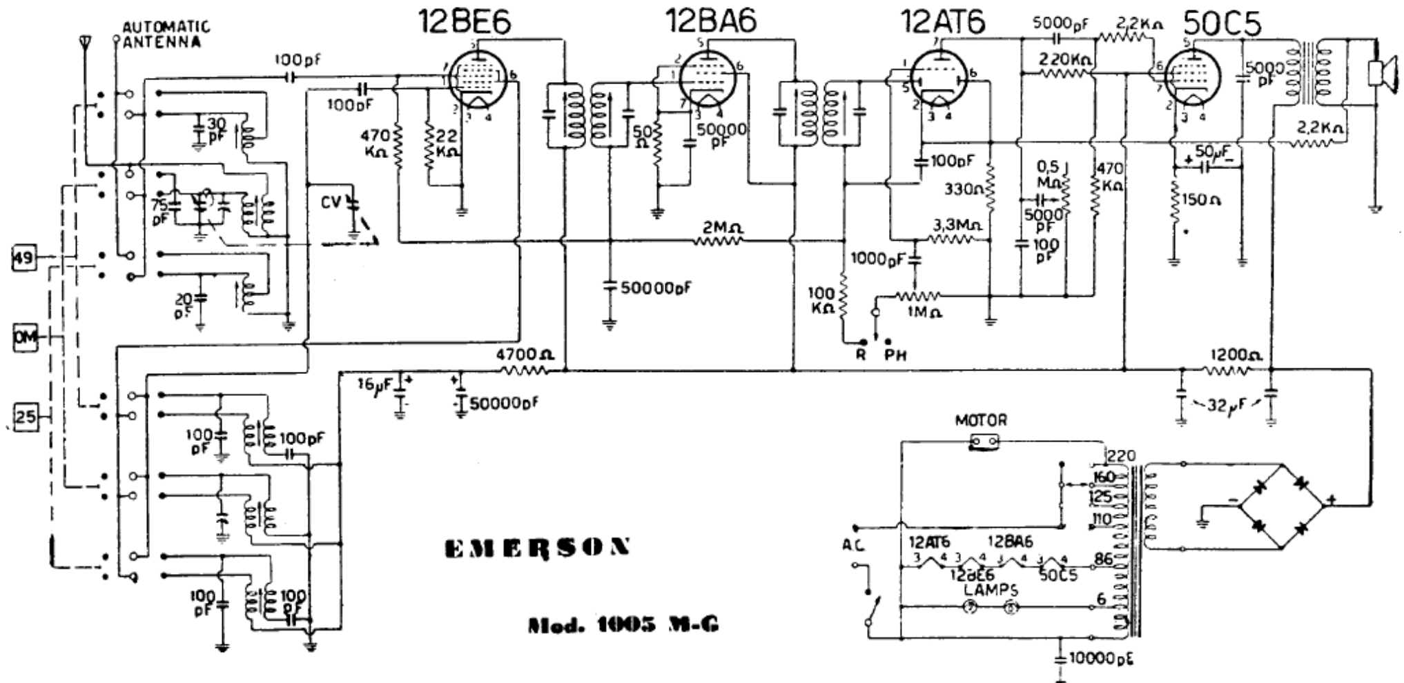
SICART-EMERSON - Mod. 1005 M-G. Onde medie e due gamme onde corte. Media frequenza 455 kc/s. Potenza d'uscita 1,5 watt. Consumo 30 watt.
